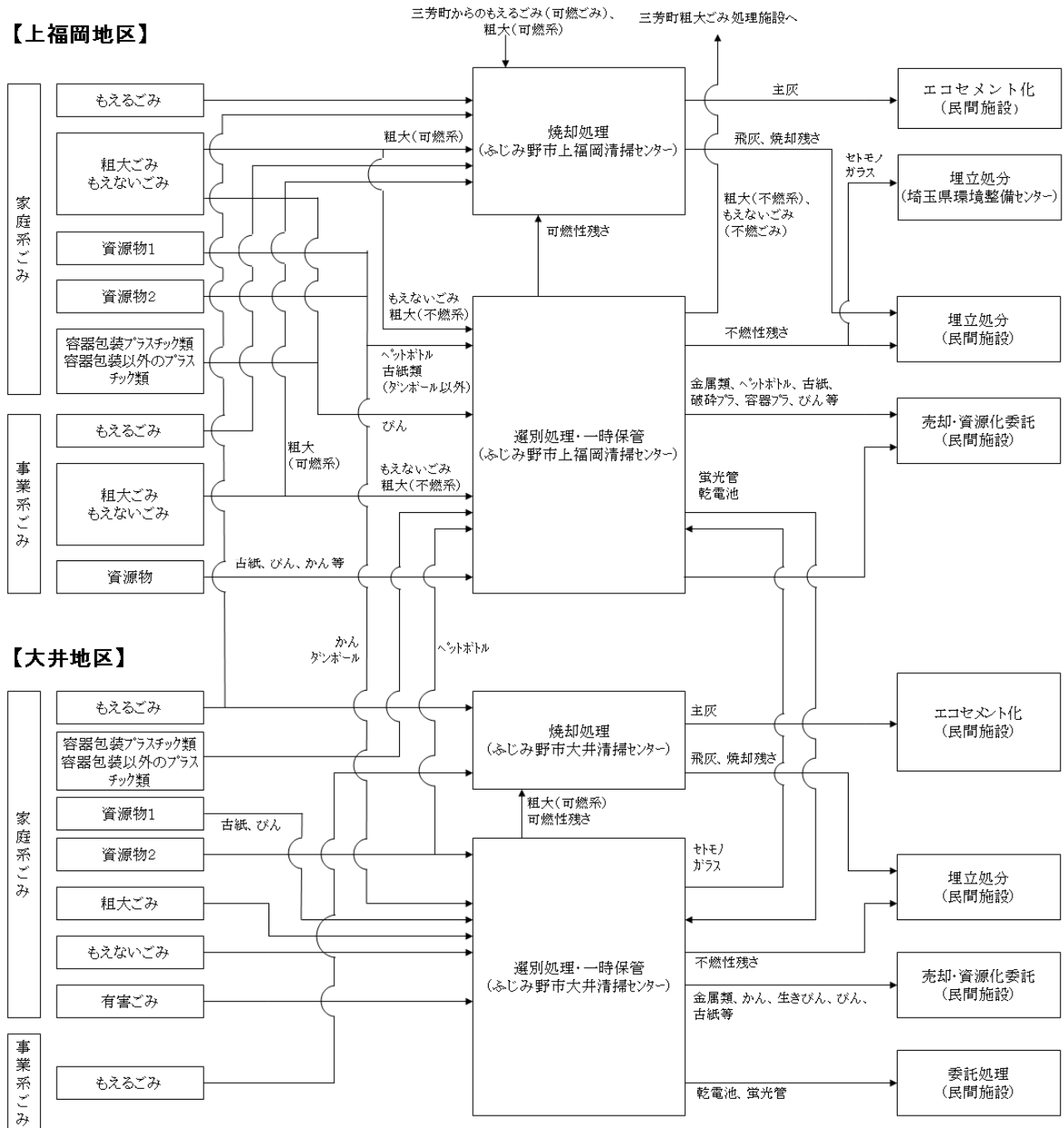
図 6-4-2 ごみ処理システム (平成 21 年度)
