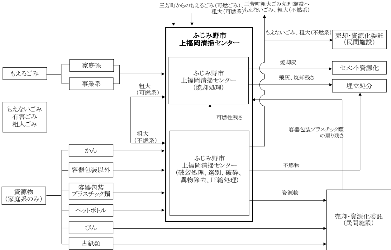
図6-4-2 ゴミ処理システム（平成24年度）
