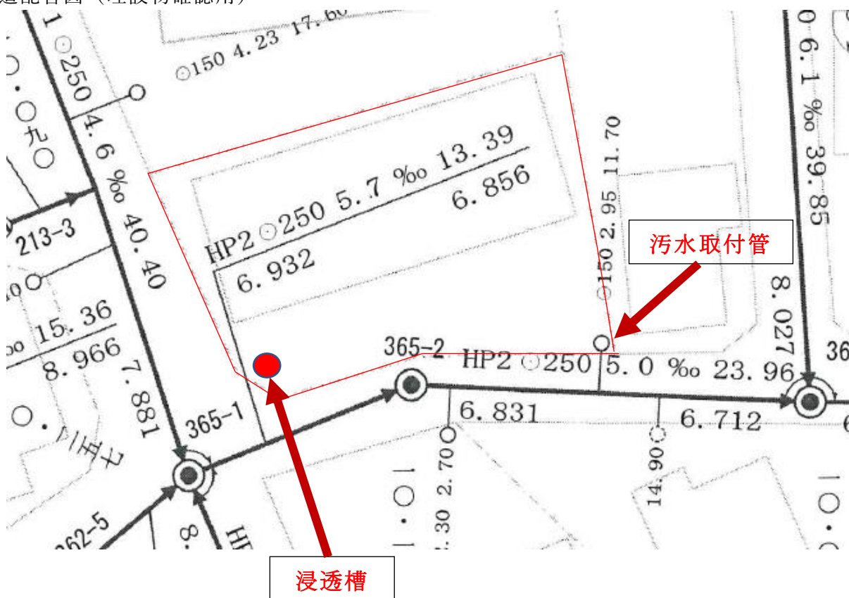
下水道配管図（埋設物確認用）
