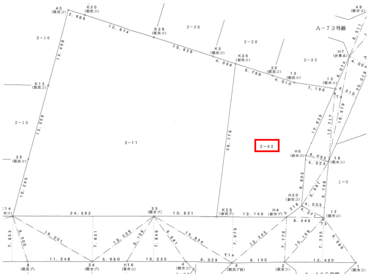
測量図
